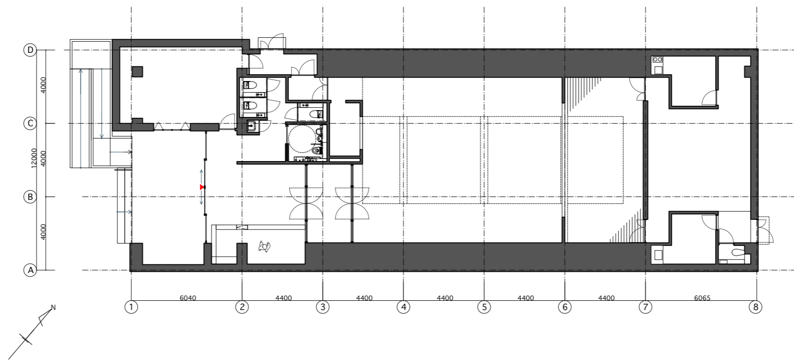
1F平面图
