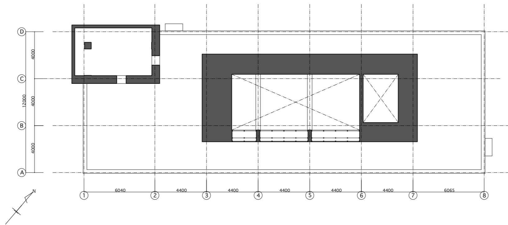
吹拔平面图
