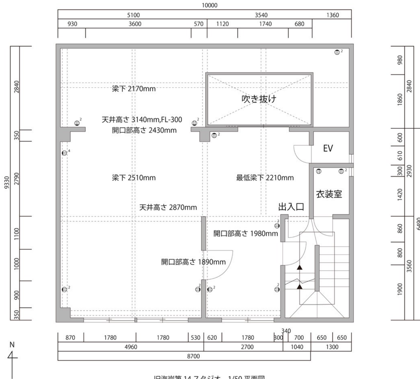
旧海岸第 14 スタジオ 1/50 平面図
